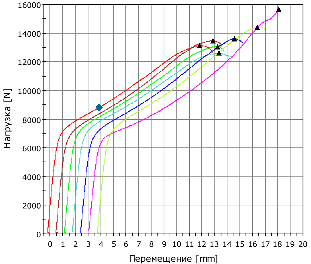
Рис. 1. Зависимость нагрузки от перемещения для образцов 1÷7
