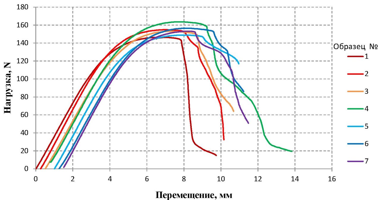
Рисунок 1. Зависимость нагрузки от перемещения для образцов REC PLA.1-7
